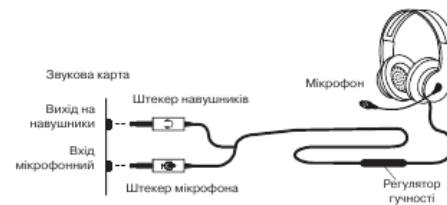
Мал. 1. Схема підключення
