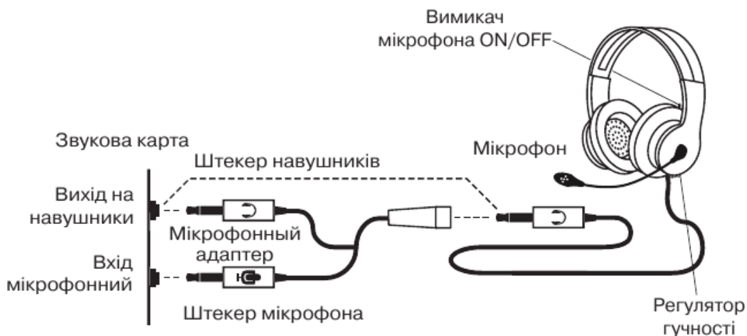
Мал. 1. Схема підключення
