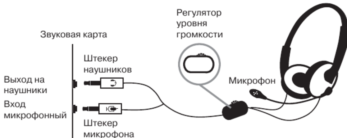
Рис. 1. Схема подключения
