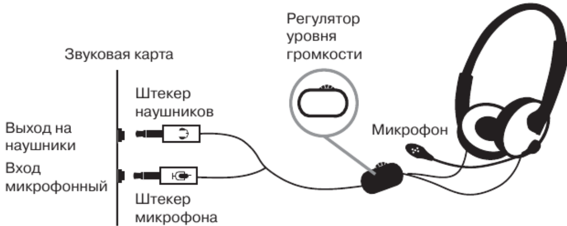
Рис. 1. Схема подключения
