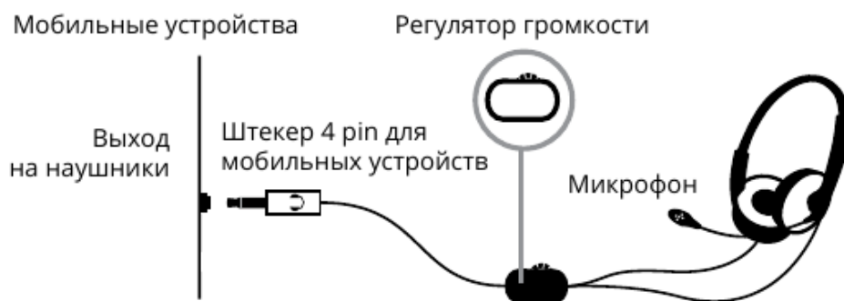
Рис. 1. Схема подключения
